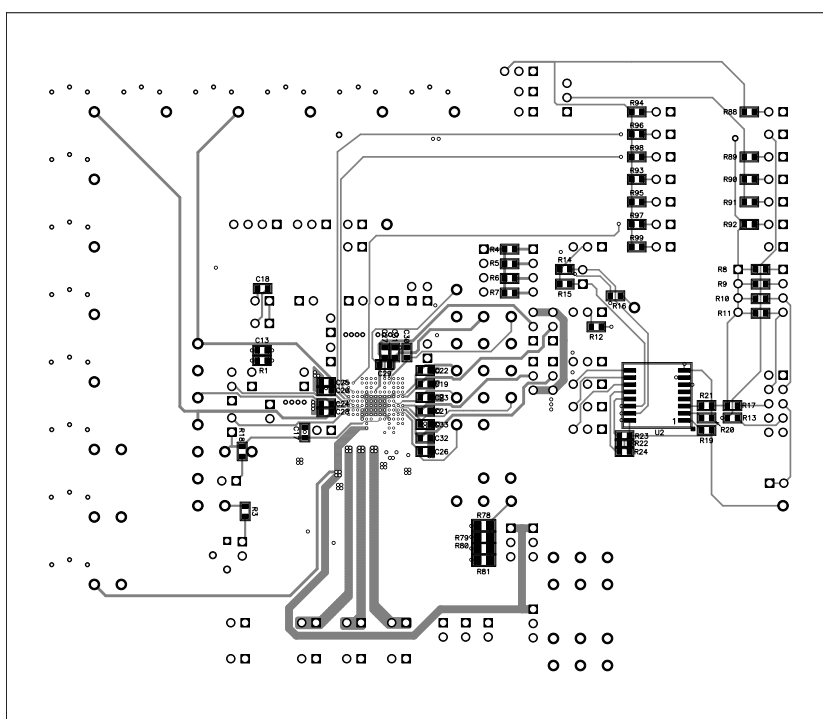
Figure 19. Bottom Layer
